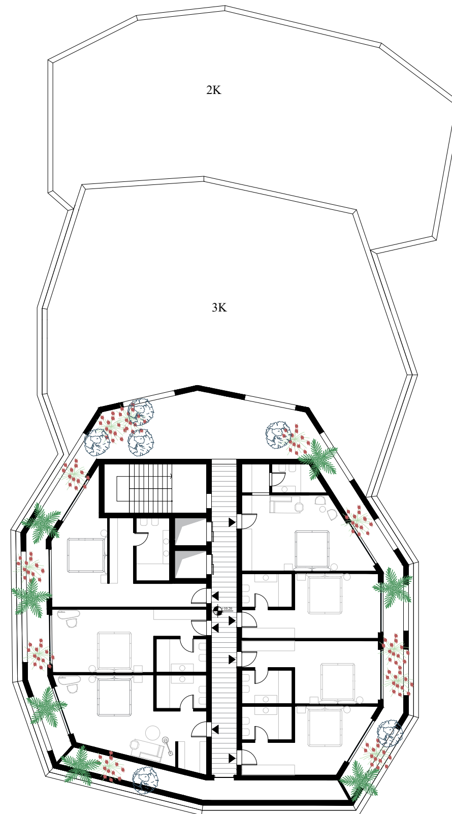
Planimetri Kati 3 / S=485.66m 2
